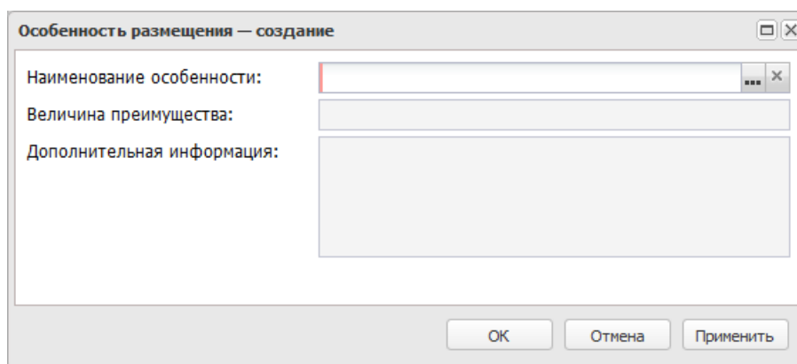
Рисунок 15 – Редактор особенностей
