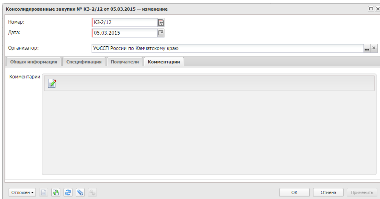
Рисунок 18 – Закладка «Комментарии»
