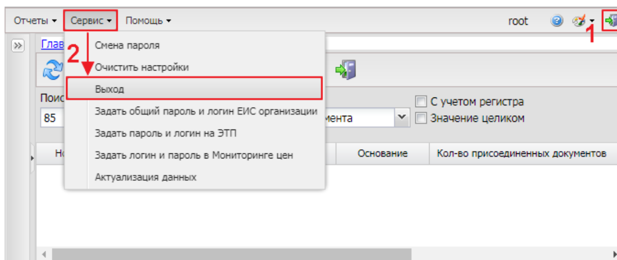
Рисунок 31 – Завершение работы
