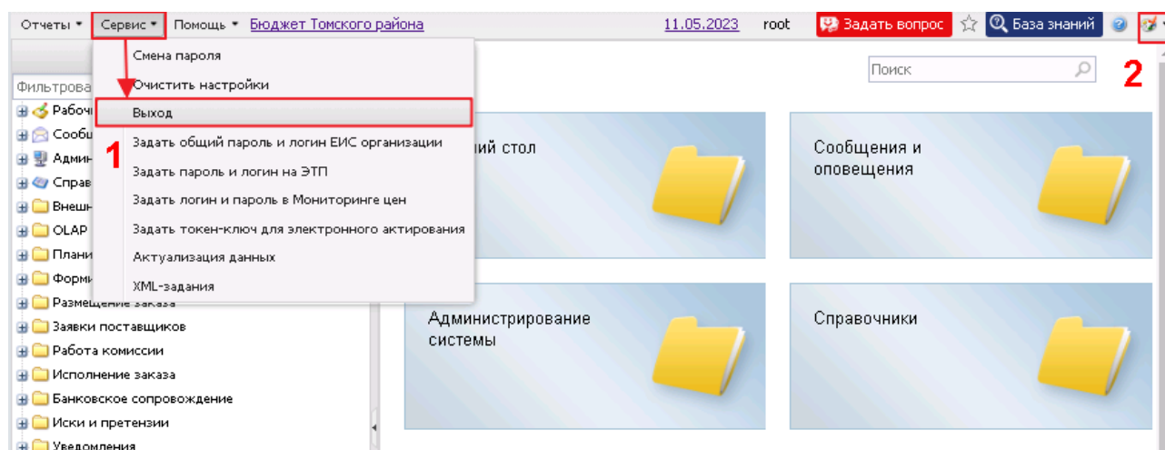
Рисунок 86 – Завершение работы
