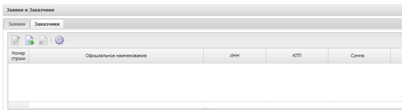
Рисунок 21 – Закладка «Заказчики»
